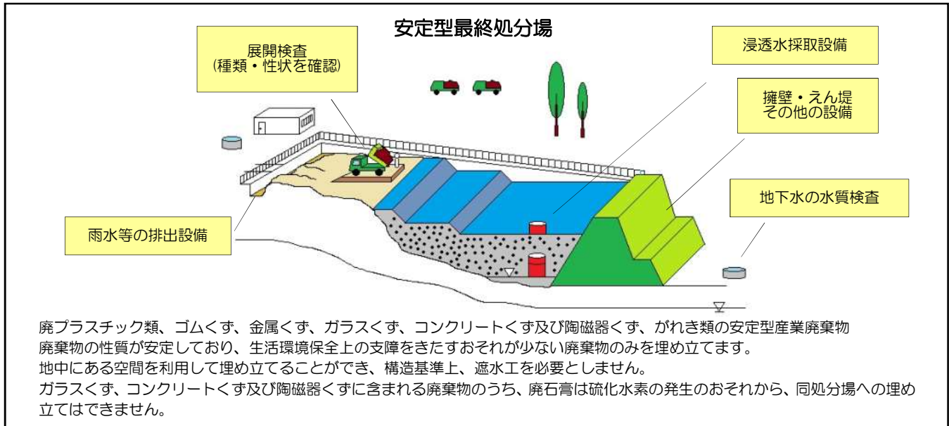
図2 管理型最終処分場の模式図 (整備を計画中)
