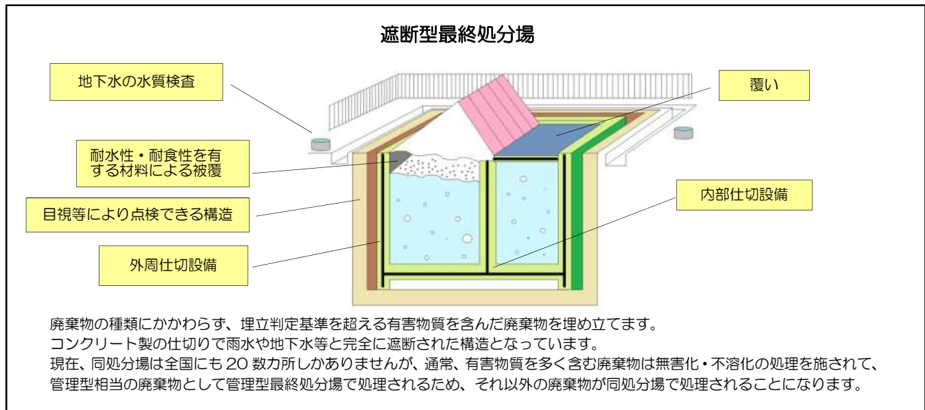
図3 遮断型最終処分場の模式図
